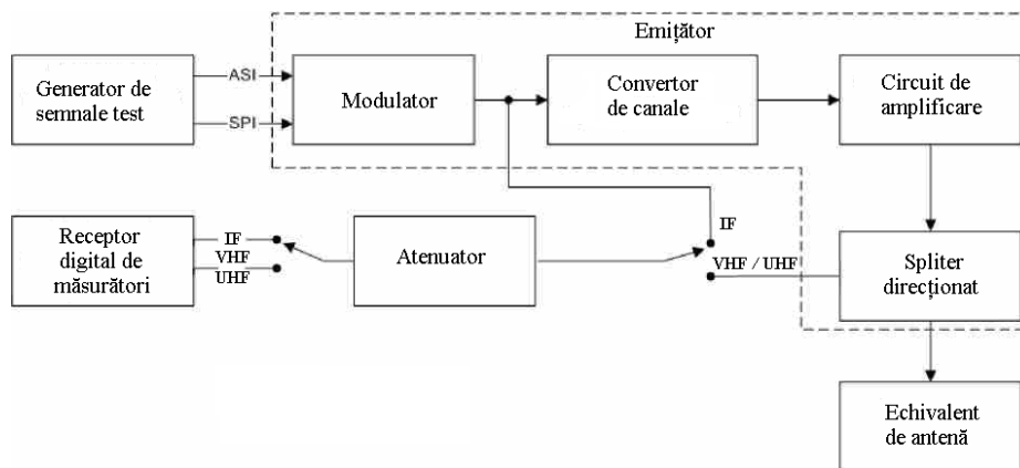
Figura 6.2.2. Schema măsurării zgomotelor echivalente ale pierderilor tractului de amplificare al emițătorului
