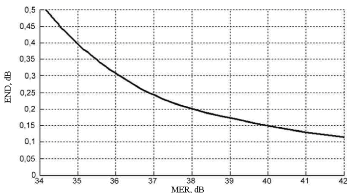
Figura 6.2.4. Dependența END de MER la distorsiuni minime
