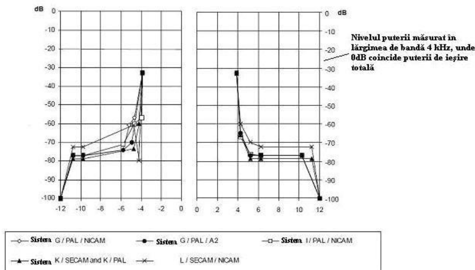
Figura 4.1.2. Măștile spectrale de protecție
