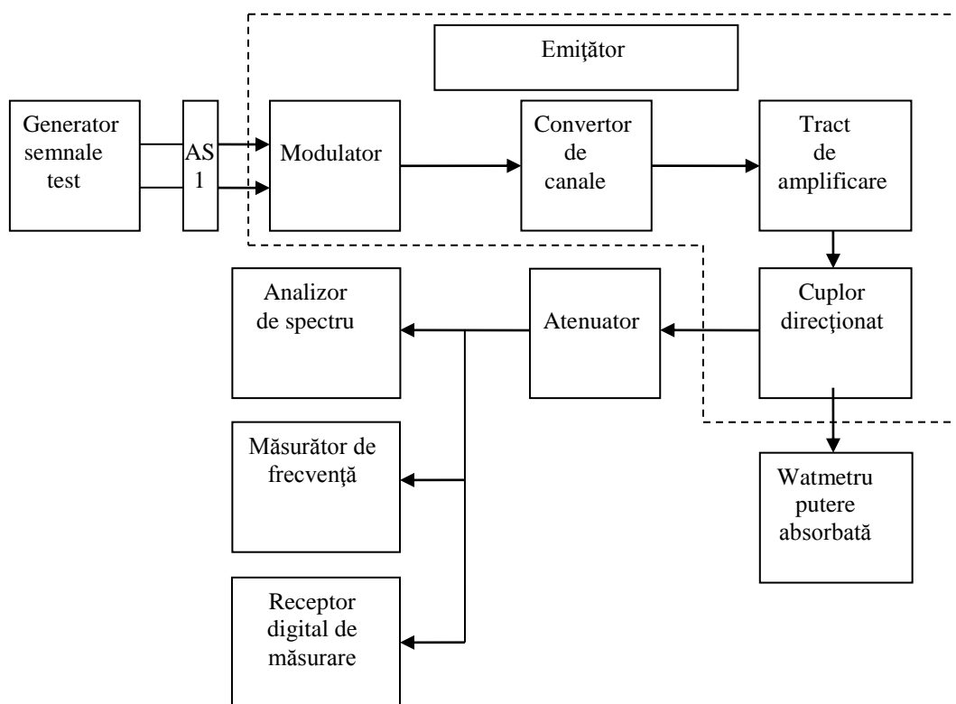
Figura 6.2.1. Schema măsurării parametrilor de bază ai emițătorului
